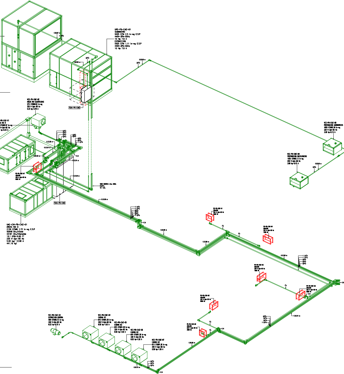
2 ISOMÉTRICO RED DE ALIMENTACIÓN 8vo. Nivel ESCALA:
